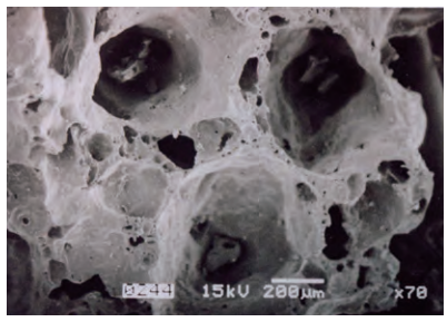
写真3-1 クリスタルバイオ(浮上タイプCB)の顕微鏡写真 撮影: 佐賀大学 (FE-SEM)×70
